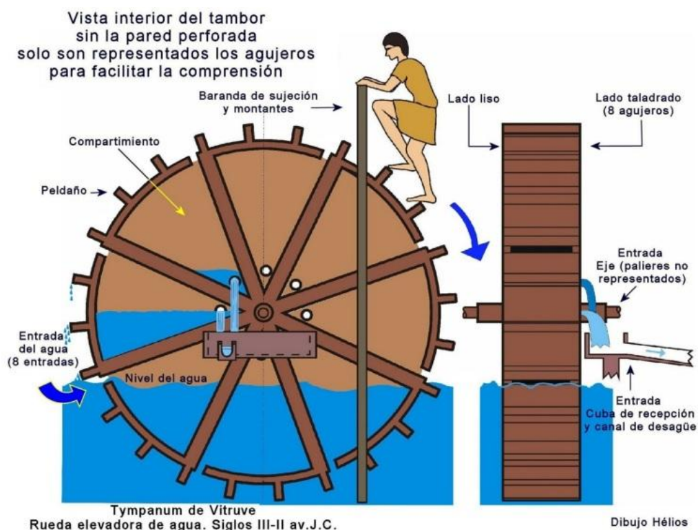
Ilustración 12. Tambor (tympano). Fuente: infraestructurasromanaspruebaticum.wordpress.com
