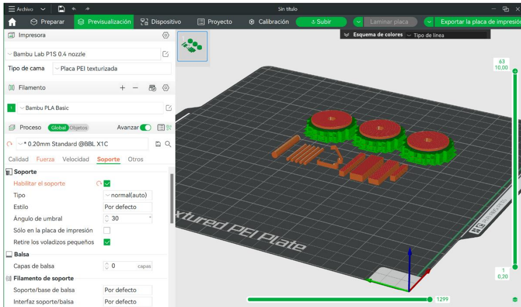
Ilustración 54. Simulación de impresión. Fuente: Elaboración propia.
