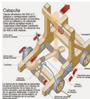
Ilustración 15. Catapulta de torsión. Fuente: pelandintecno.blogspot.com
