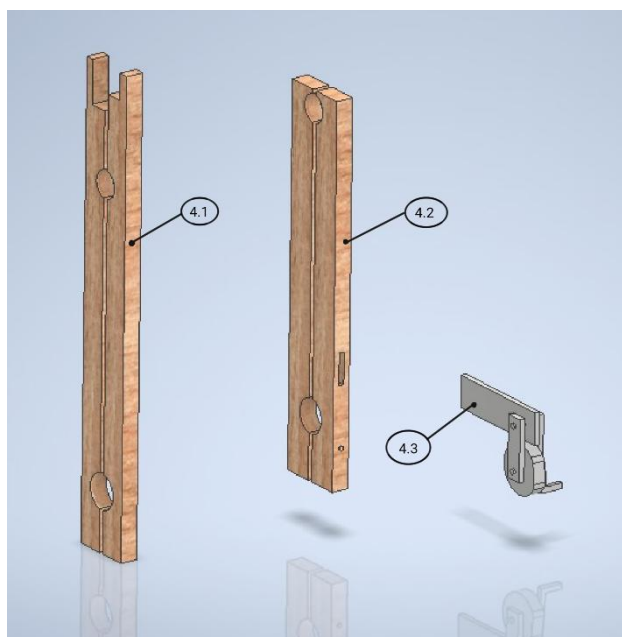
Ilustración 28. Subconjunto 4: Soporte de rueda. Fuente: Elaboración propia.
