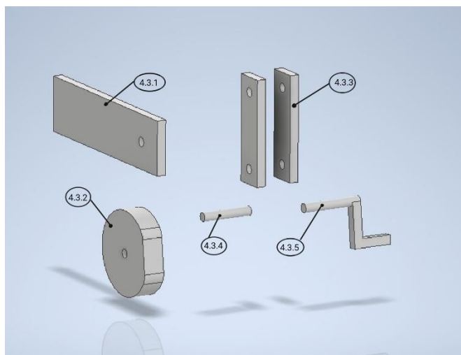
Ilustración 29. Subconjunto 4.3: Freno. Fuente: Elaboración propia
