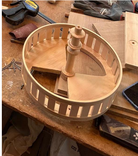
Ilustración 58. Rueda ensamblada. Fuente: Elaboración propia
