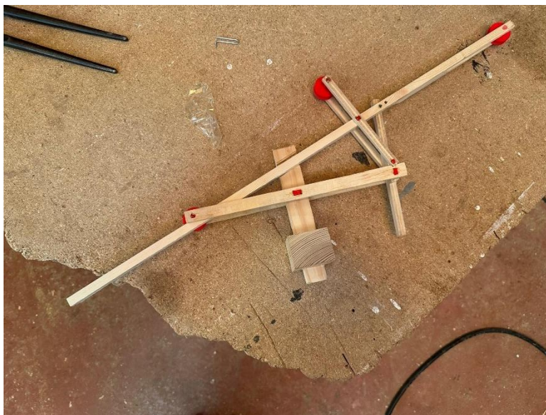
Ilustración 56. Esqueleto móvil ensamblado. Fuente: Elaboración propia
